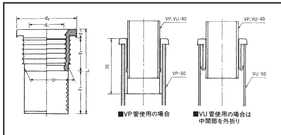
UL-45 断面図・取付図
